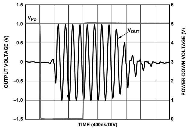
Figure 27. Enable/Power-Down Time
